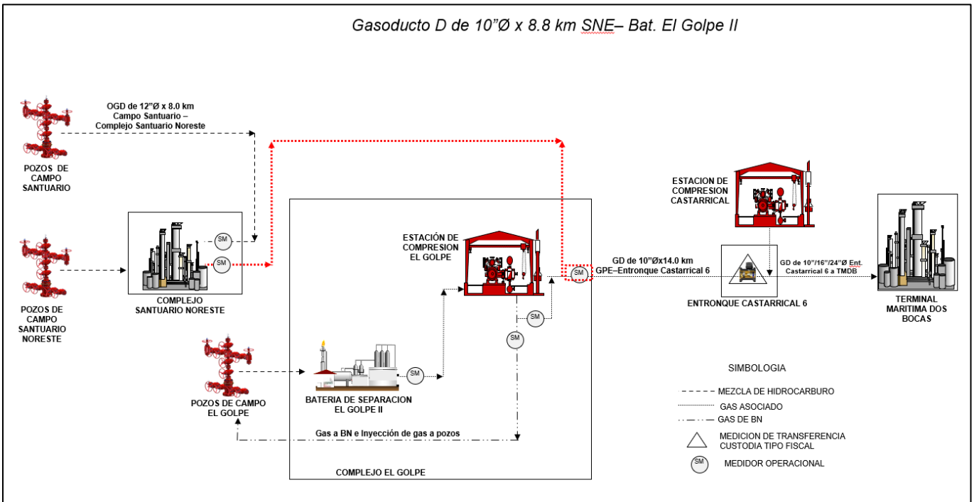
Figura 3. Diagrama esquemático de procesos – Oleoducto 10" Ø de 8.8 Km SNE-Complejo Golpe
