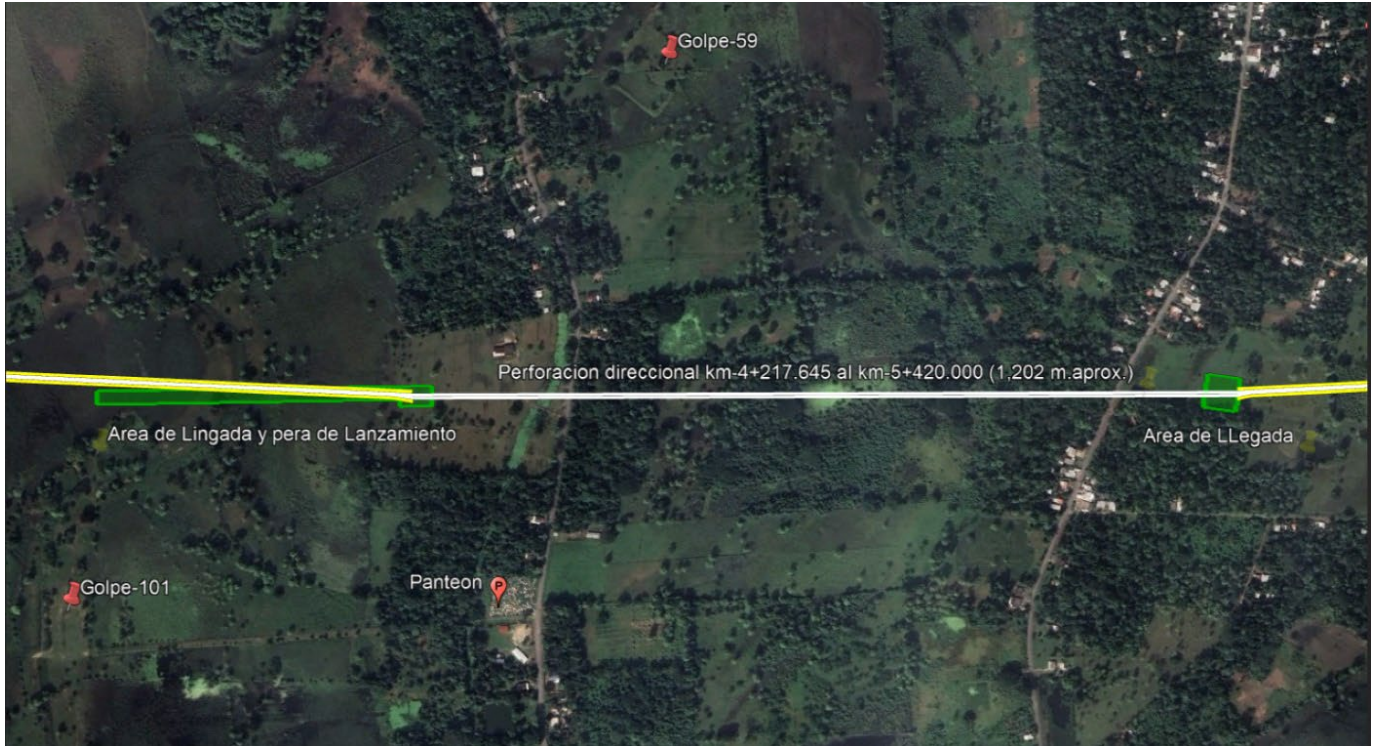
Figura A.3. Direccional: del km 4+217.645 al km-5+445.085
